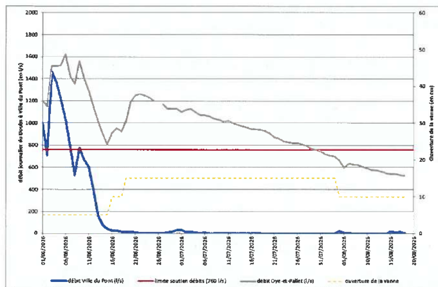
Figure 4 Comparaison entre les débits à la sortie du Lac (Oye-et-Pallet) et Ville du Pont
