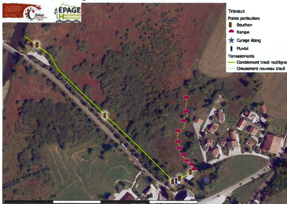
Figure 2 Plan général des travaux
