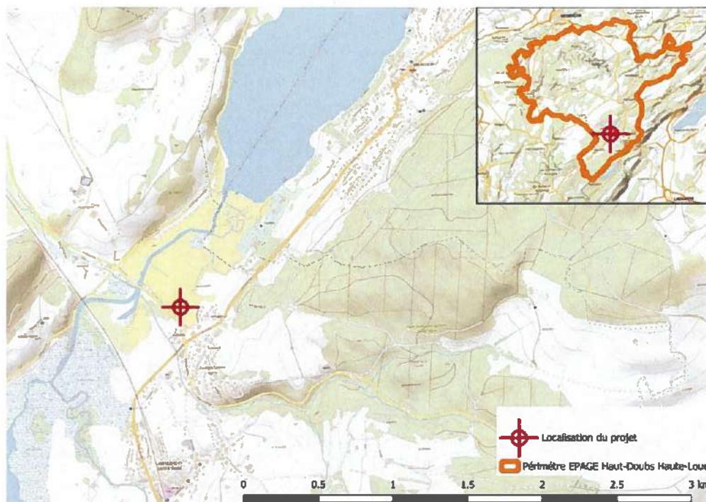
Figure 1 Localisation générale du projet (fond SCAN 1000 – IGN)
